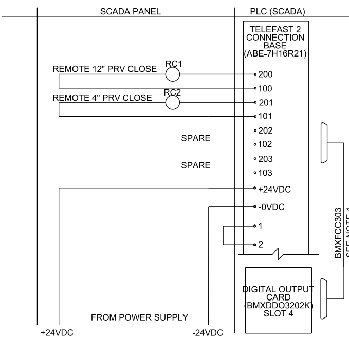
B SCADA DIGITAL OUTPUT SCALE: N.T.S.
