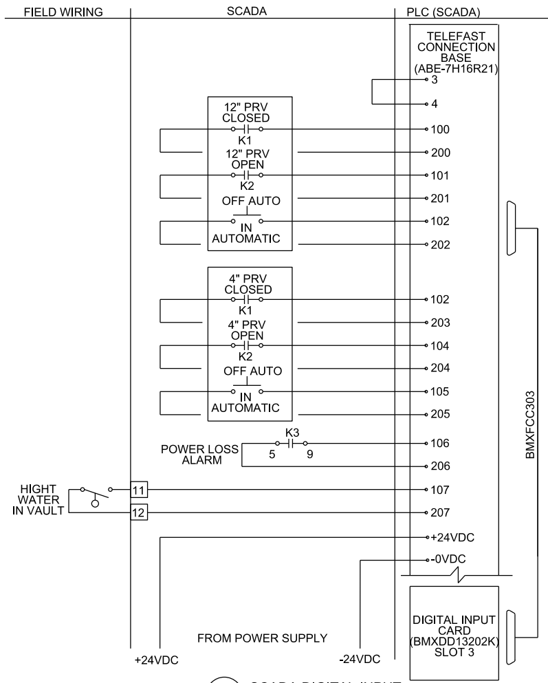
A SCADA DIGITAL INPUT SCALE: N.T.S.
